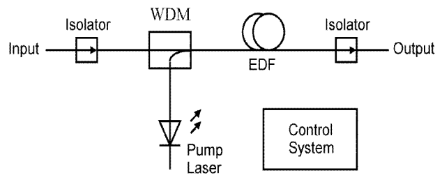
Fig. 1. EDFA Scheme
